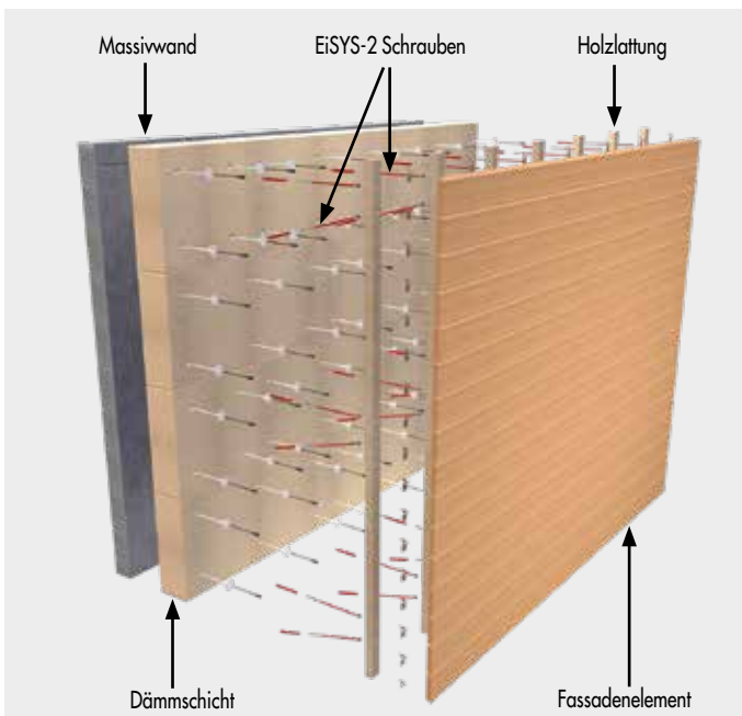
EiSYS-2 zur Befestigung einer horizontalen Holz-Unterkonstruktion, durch Dämmstoff in eine Betonaußenwand.
