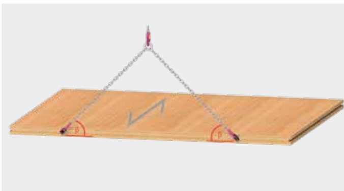
BSH-Wand oder-Träger liegend, Faserverlauf: vertikal
