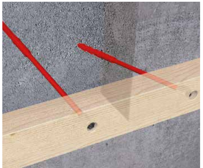
EiSYS-2 zur Befestigung einer horizontalen Holz-Unterkonstruktion, durch Dämmstoff in eine Betonaußenwand.
