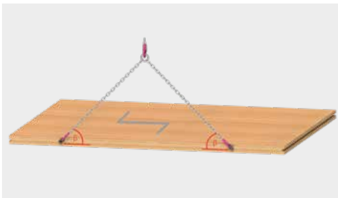
BSH-Wand oder-Träger liegend, Faserverlauf: horizontal
