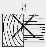
Querzugverstärkung an Auskinkung
