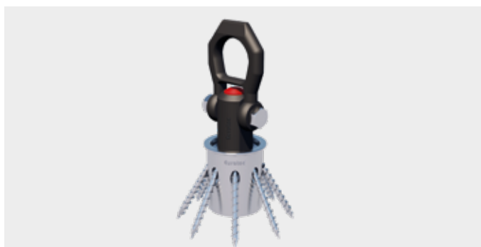
Der Hebeanker HebeFix Mini in Kombination mit dem Kugeltragbolzen.
