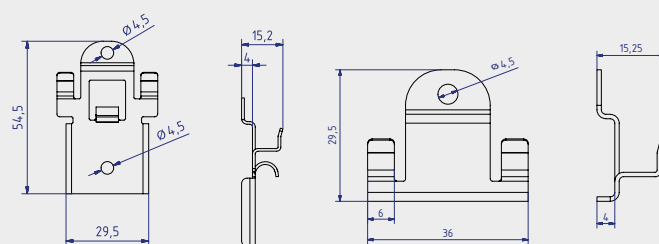
Fassadenclip-Rhombus
