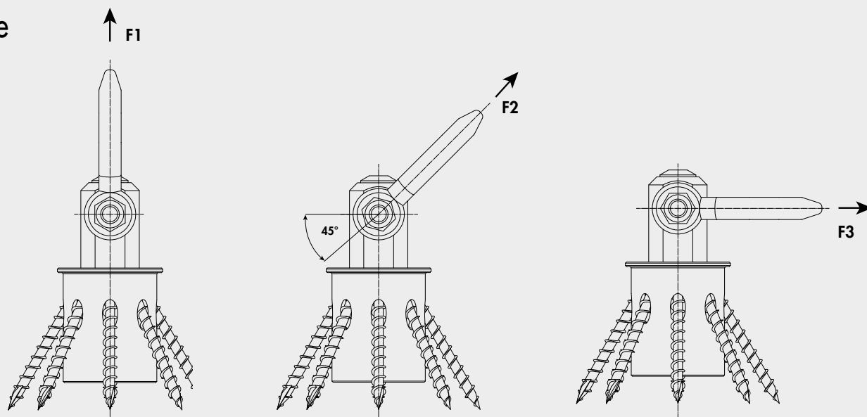
Der Hebeanker HebeFix Mini in Kombination mit dem Kugeltragbolzen.
