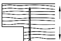
Querzugverstärkung an Auskinkung
