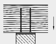
Auflagerverstärkung
