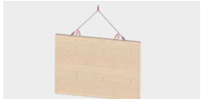
CLT-Wand oder-Träger stehend
